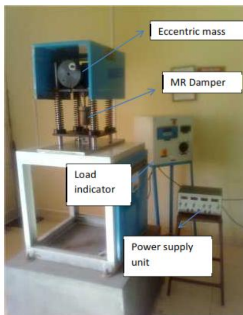
Fig. 4.1 MR Damper test rig.
